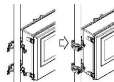
図1: 単管クランプによる固定
